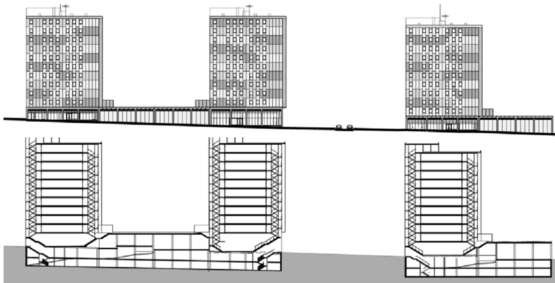
Alçats i seccions.
