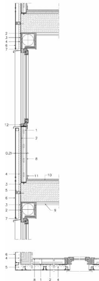
Secció façana.
