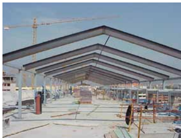
Estructura sotacoberta.
